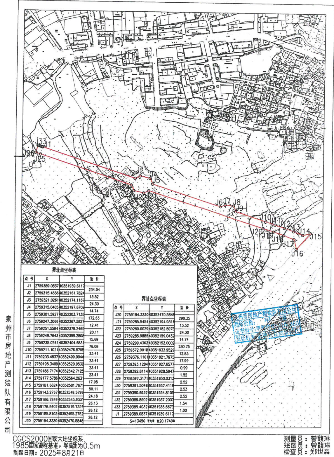
华星路市政道路工程勘测定界图
